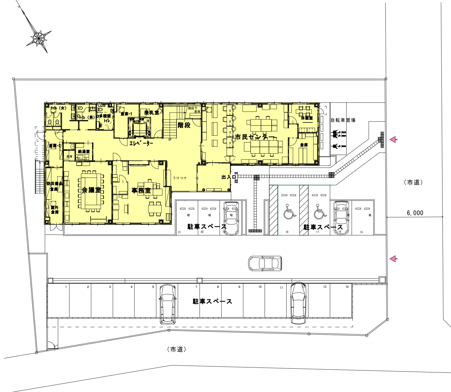
配置図・1階平面図
